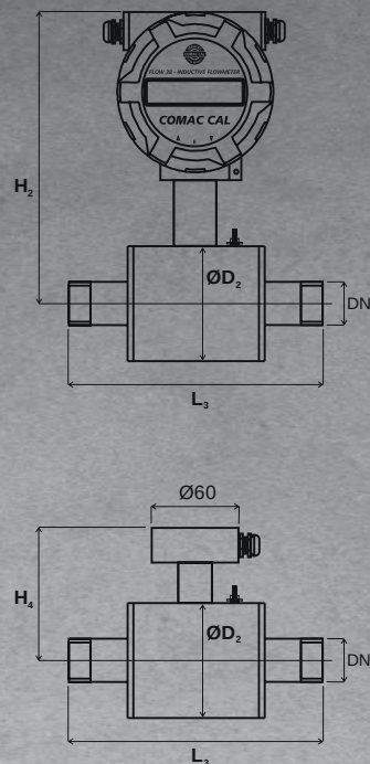
THREAD (EN 10226-1)
